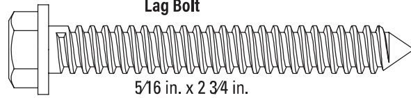
Lag Bolt
