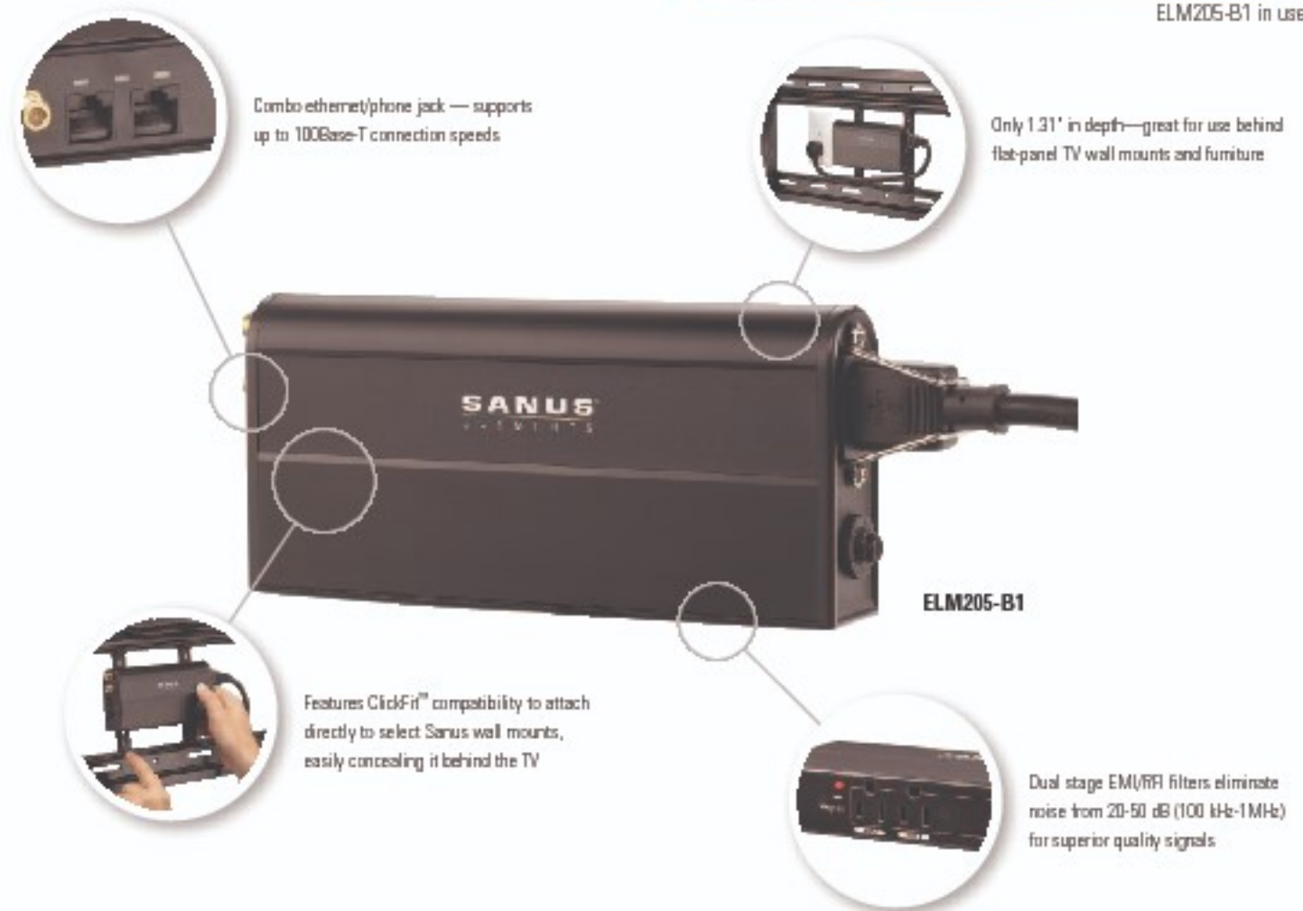
ELM205-B1 in use
